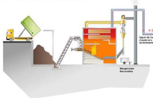
Synoptique fonctionnement chaufferie bois
